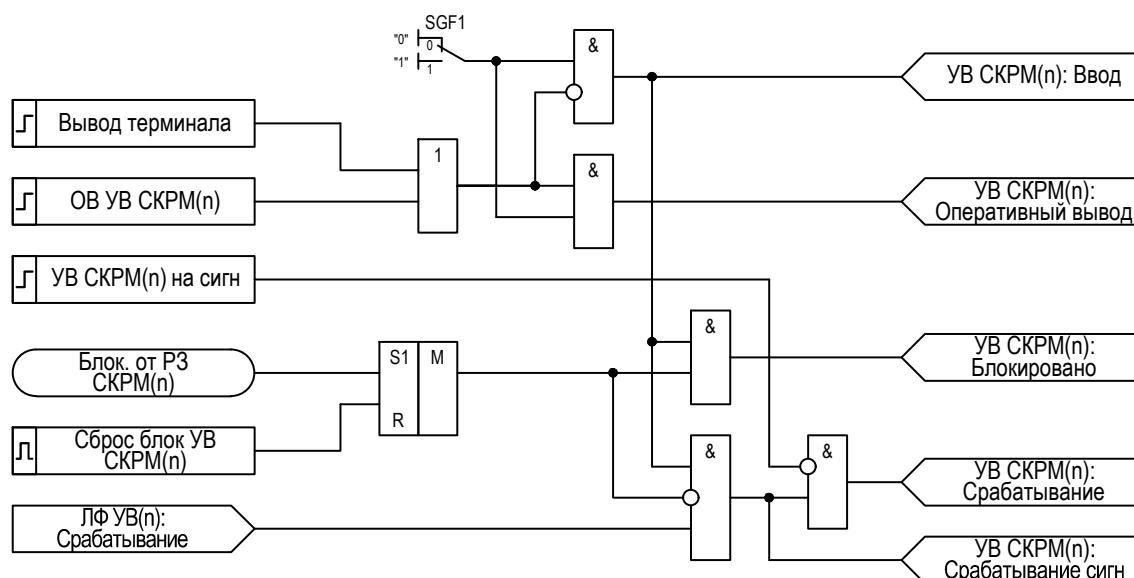
Рисунок 2.20 – Функциональная схема УВ СКРМ
