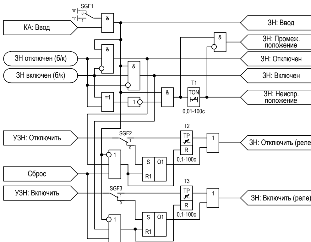
Рисунок 2.26 – Функциональная схема «ЗН»
