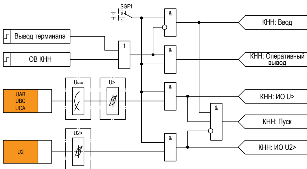
Рисунок 2.22 – Функциональная схема «КНН»
