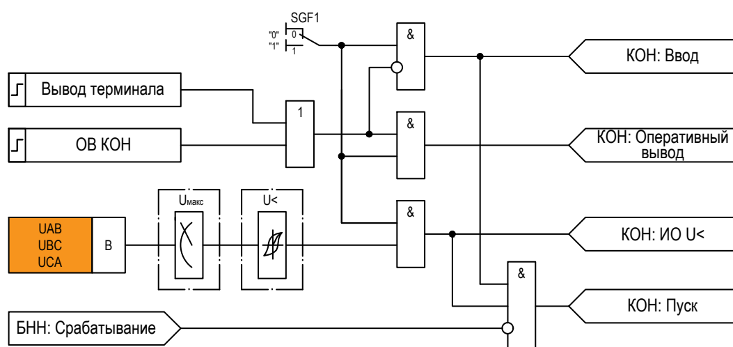
Рисунок 2.23 – Функциональная схема «КОН»
