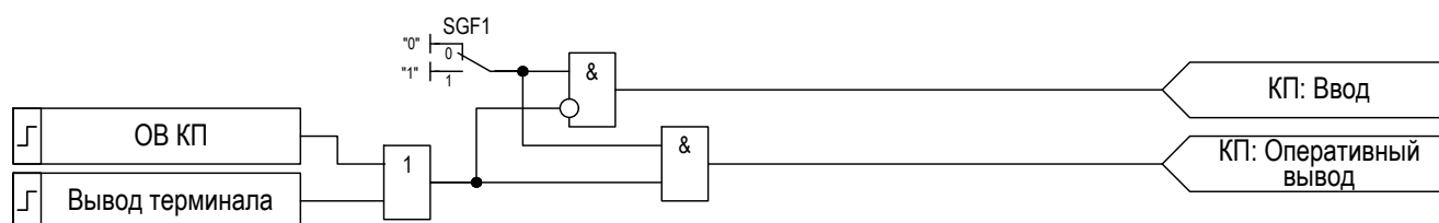
Рисунок 2.28 – Функциональная схема управления режимами работы функционального блока «КП»
