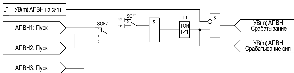
Рисунок 2.8 – Функциональная схема «УВ(м) АПВН»
