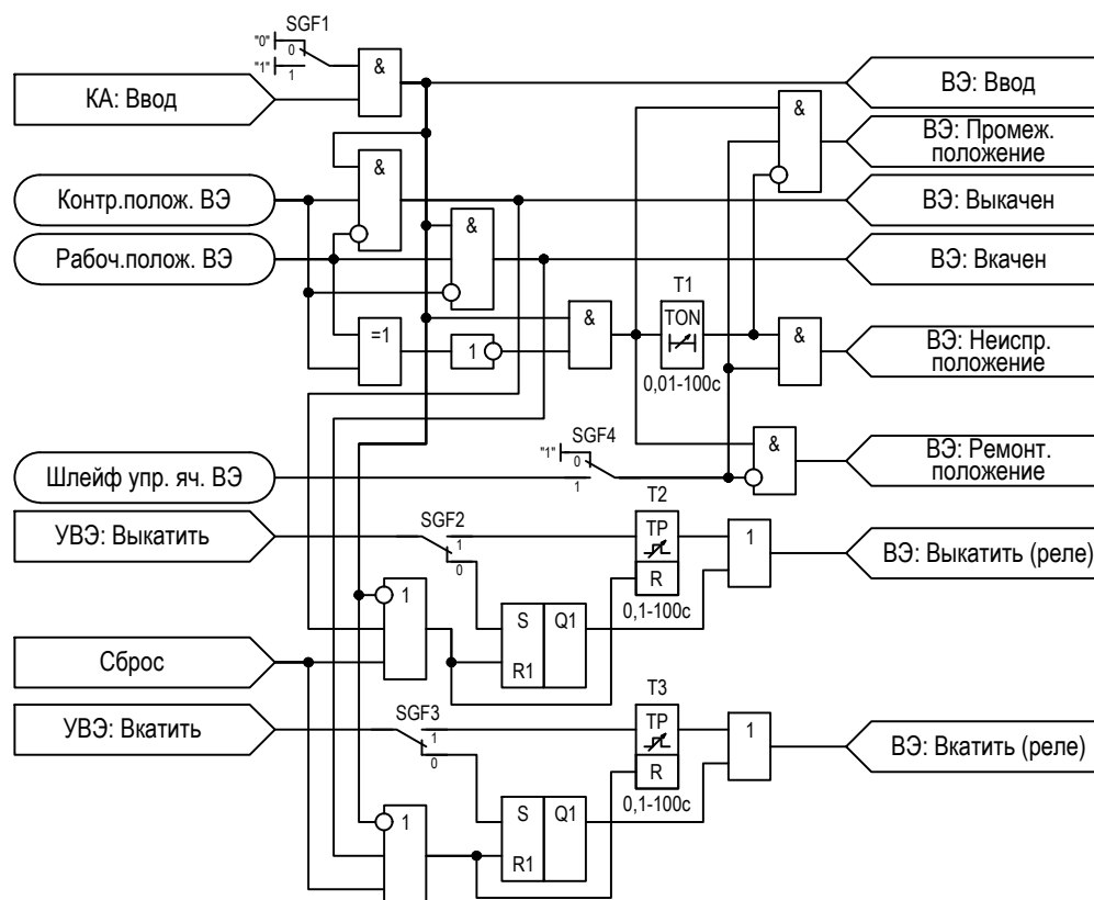
Рисунок 2.27 – Функциональная схема «ВЭ»
