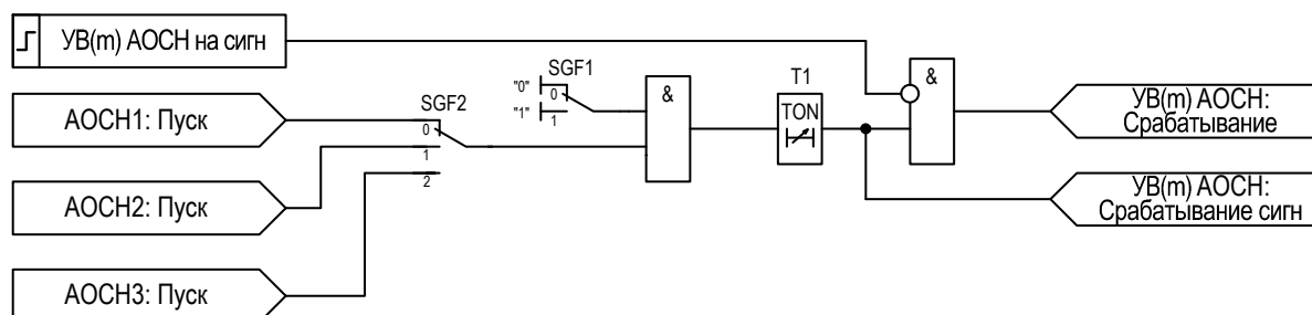
Рисунок 2.6 – Функциональная схема «УВ(м) АОСН»
