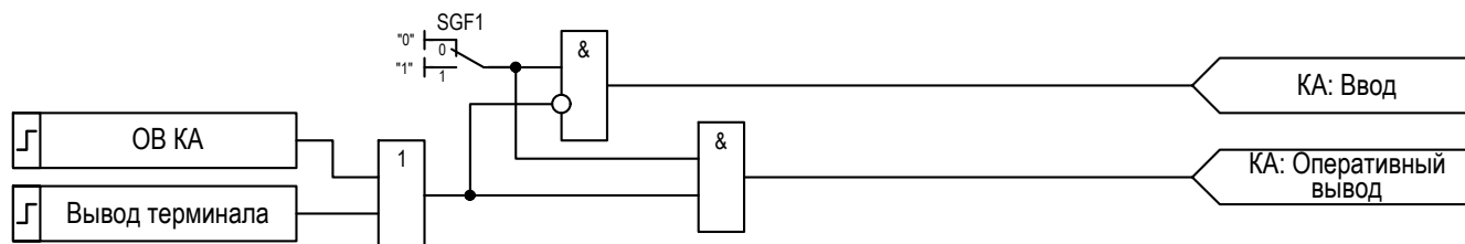
Рисунок 2.25 – Логика управления режимами функционального блока «КА»
