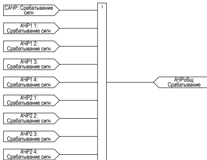
Рисунок 2.14 – Функциональная схема сборки сигналов АЧР
